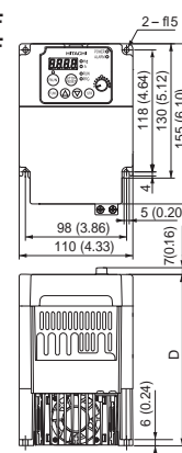
¥SJ200-007 - 022NFEF ¥SJ200-004 - 040HFEF
