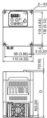
¥SJ200-007 - 022NFU ¥SJ200-030 - 037LFU ¥SJ200-004 - 037HFU
